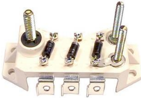
DIODETRIO 33-403 TRIO 8E SER ALT THERMO KING
